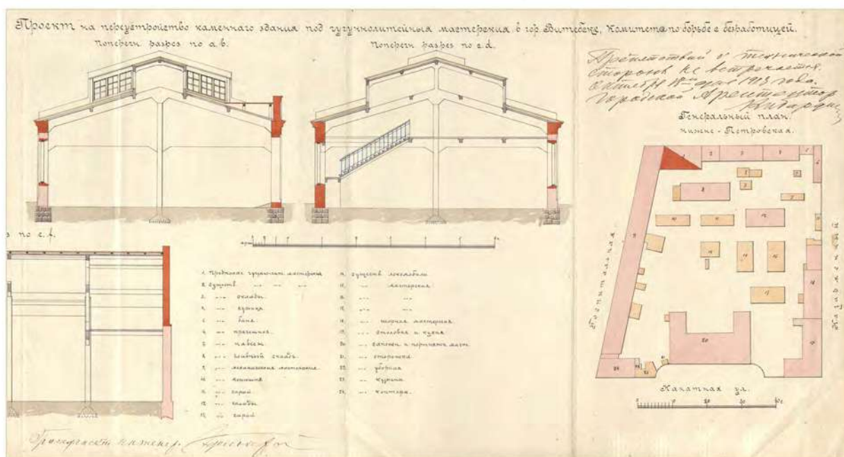
Рис. 5. Проект на переустройство каменного здания под чугунолитейные мастерские в гор. Витебске Комитета по борьбе с безработицей. Фрагмент. ГАВО. Ф. 238. Оп. 1. Д. 6. Л. 429. 1918
